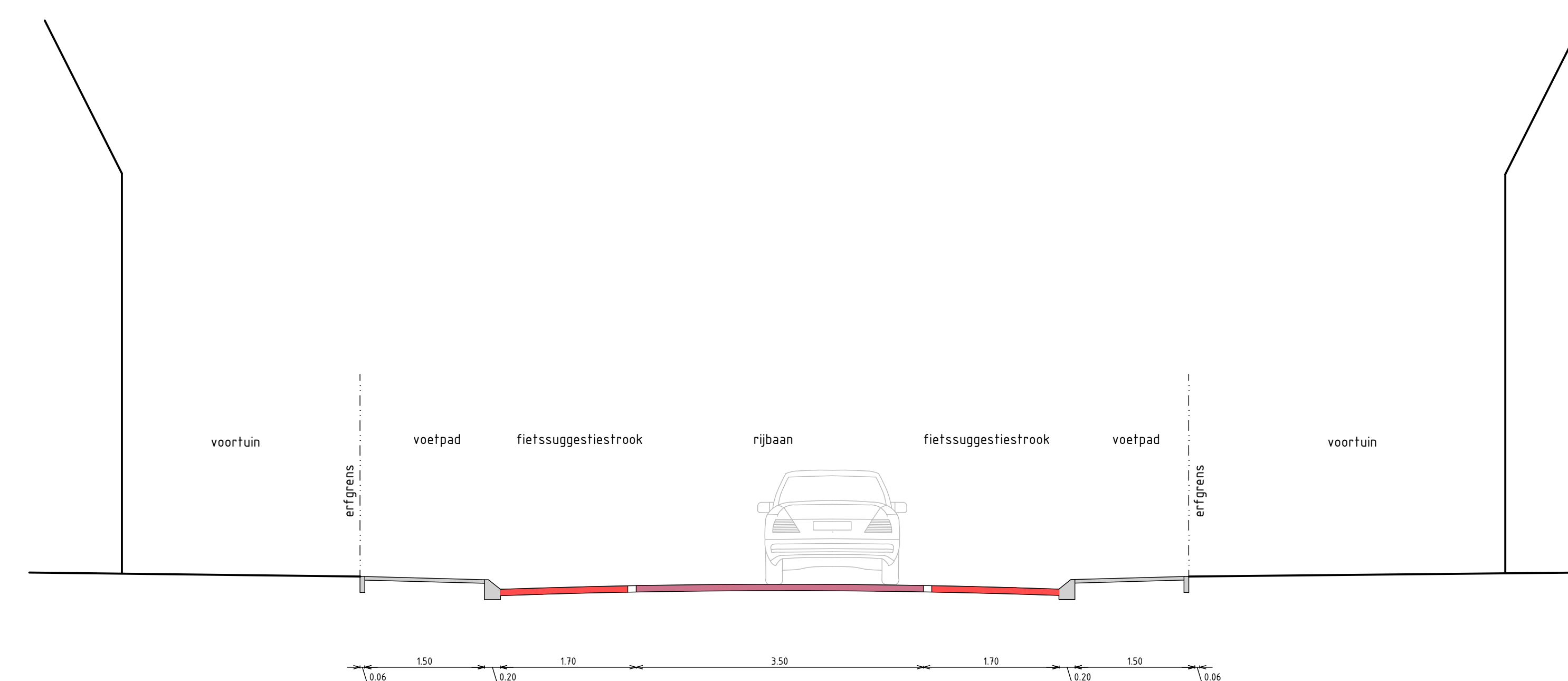
Doorsnede B-B Schaal 1:50
