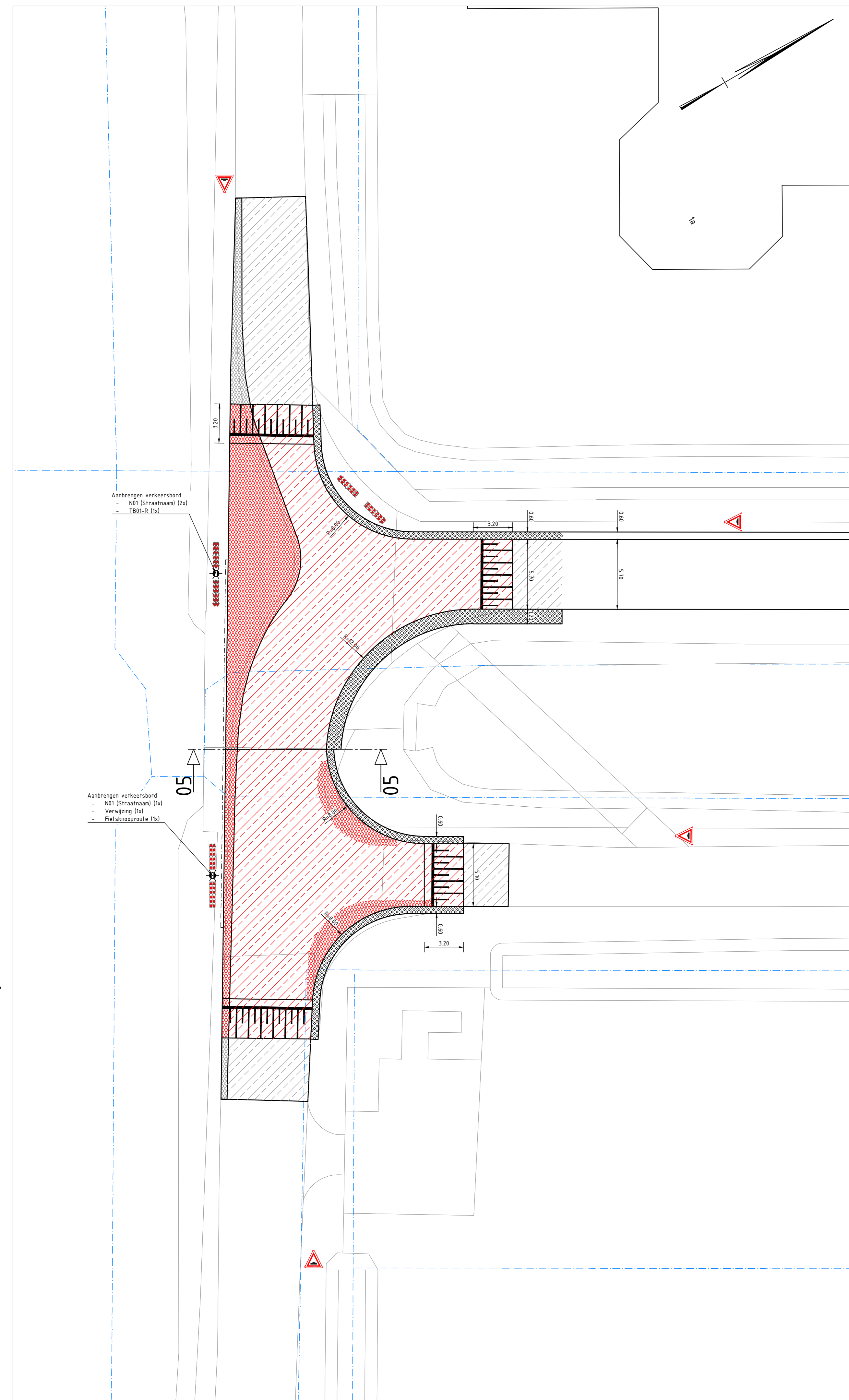
Overzicht kruising Zandvaart en Molenvaart schaal 1: 200
