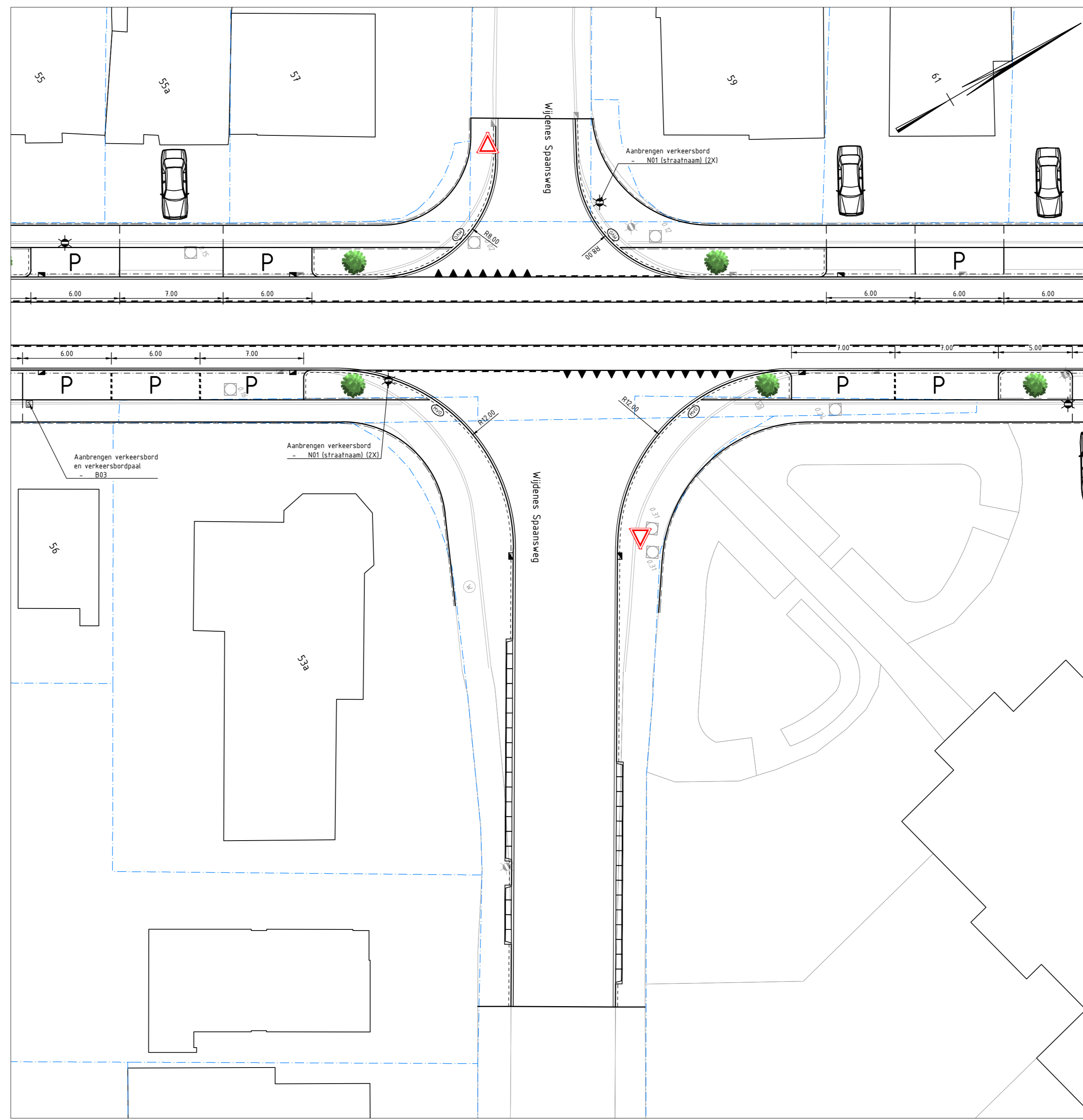
Overzicht kruising Burgemeester Lovinkstraat en Wijdenes Spaansweg schaal 1: 200
