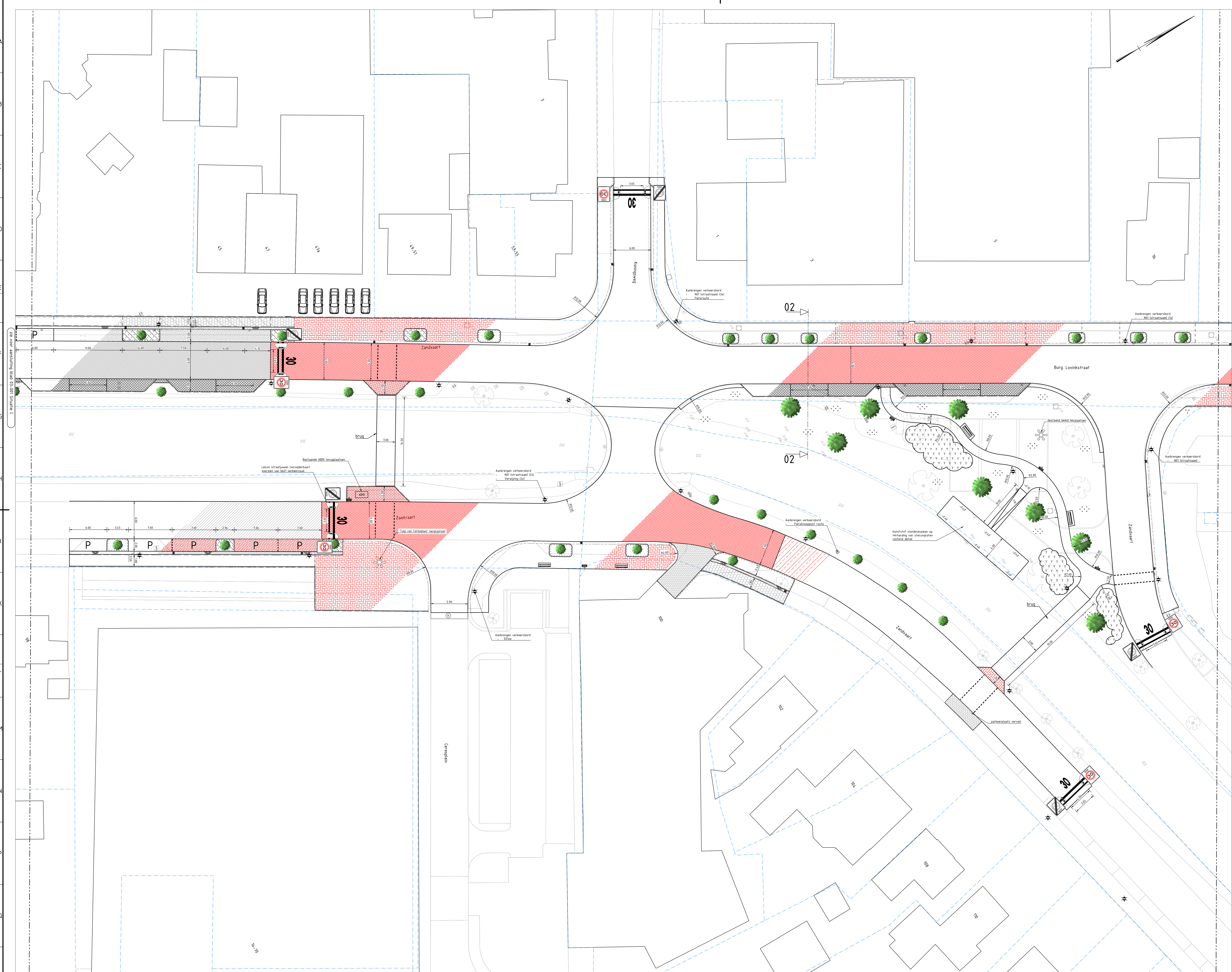
Situatie A Zandvaart (plein) schaal 1 : 200
